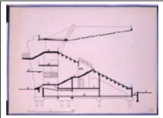
Stade municipal : coupe transversale sur la tribune, n.d. © CNAM/DAF/Cité de l'architecture et du patrimoine / Archives d'architecture du XX e siècle.
