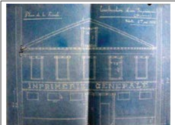
Elévation de la façade de l'imprimerie, vers 1900 AMSD, 2 O 80
